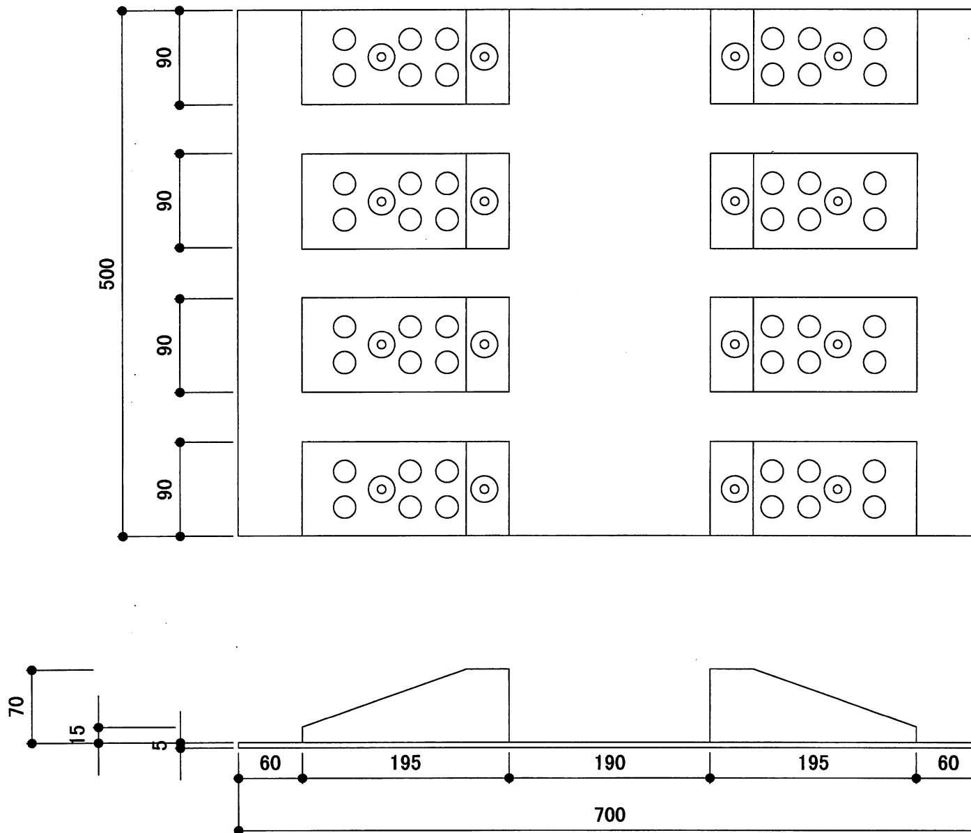
ホースブリッジ外觀図
