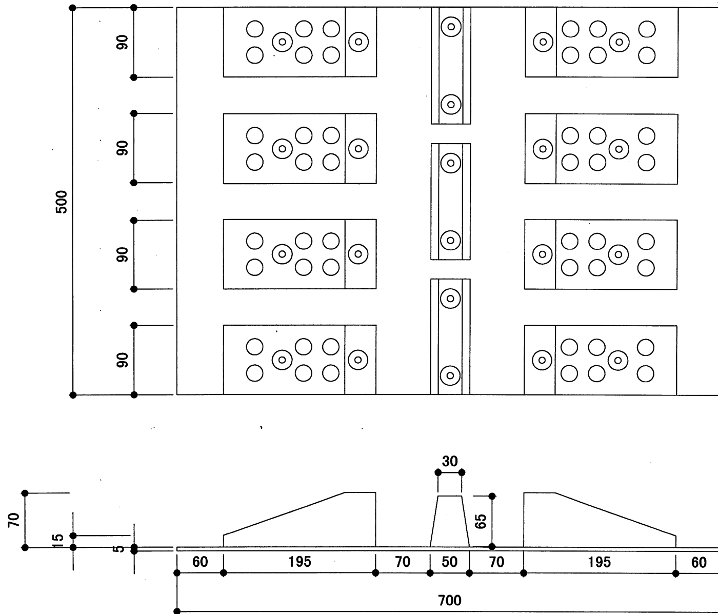
ホースブリッジ外觀図
